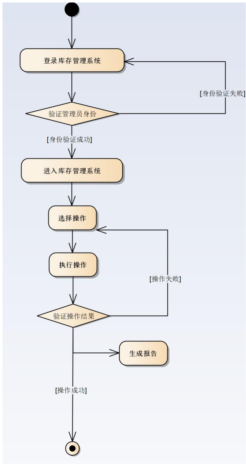
图 8.4.4 ： 库存管理 – 活动图
