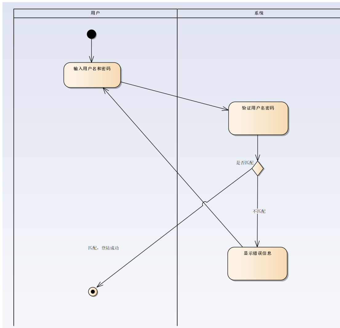
图 8.1.4 ： 用户管理 – 活动图
