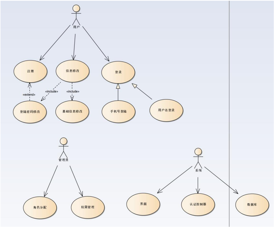
图 8.1.1 ： 用户管理 – 用例图
