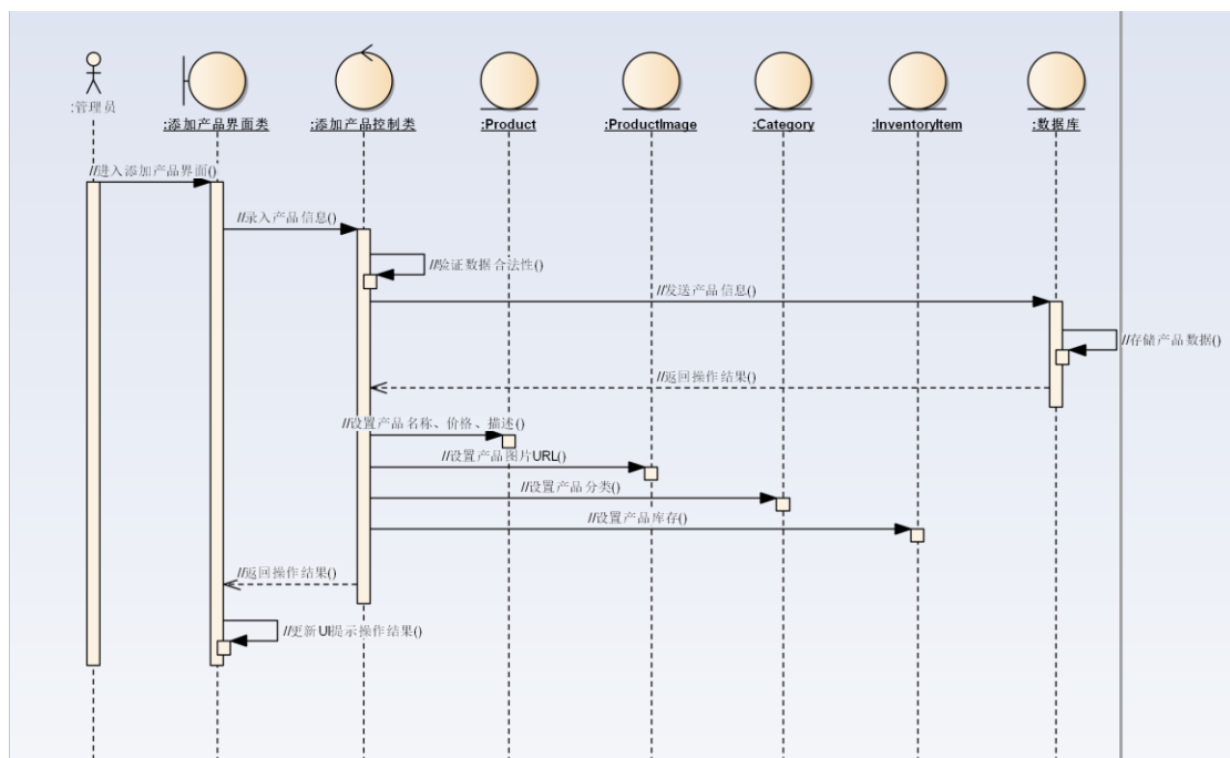
图 8.3.3 : 产品管理 – 顺序图
