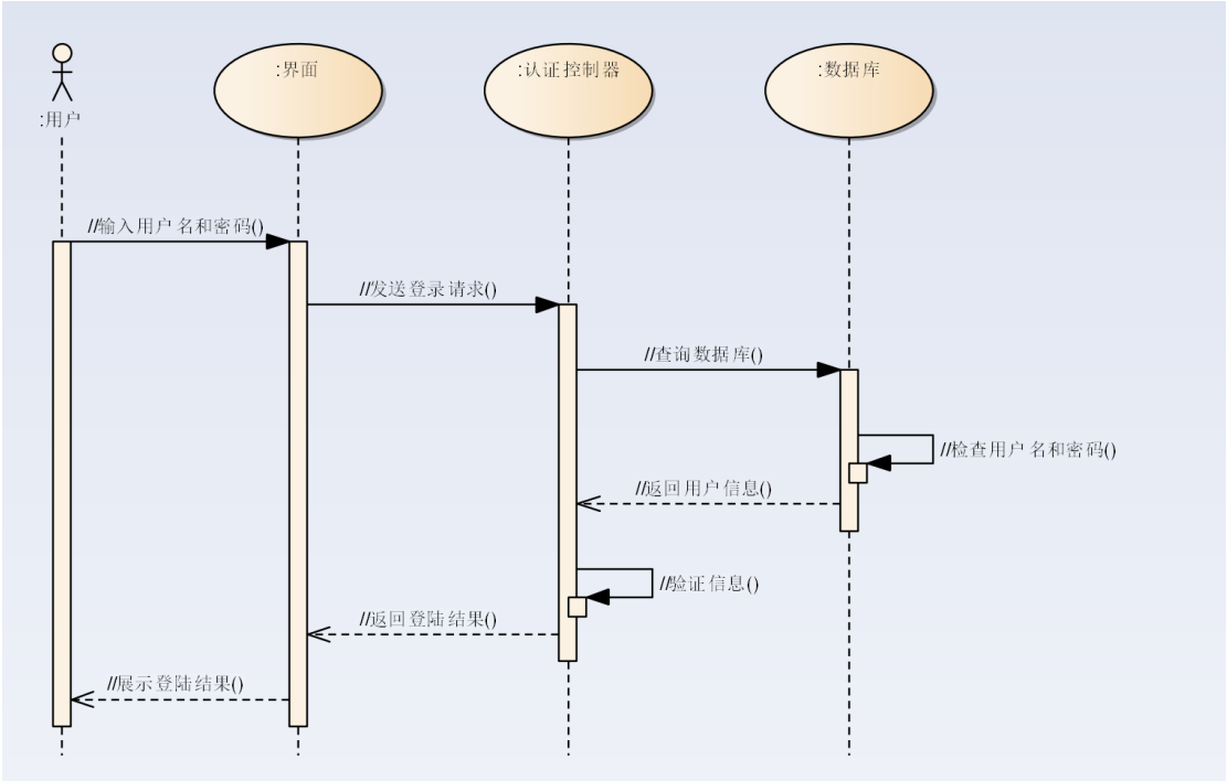
图 8.1.3 ： 用户管理 – 顺序图
