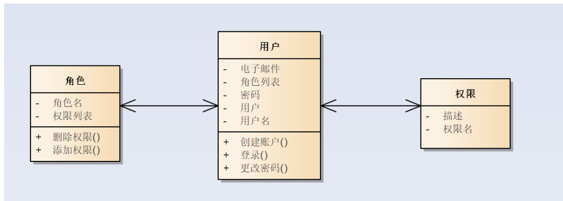
图 8.1.2 ：用户管理 – 类图
