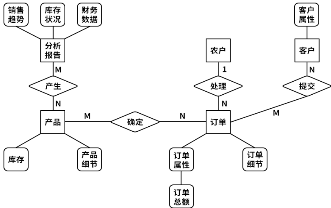
图 6.6.4.1：实体关系图
