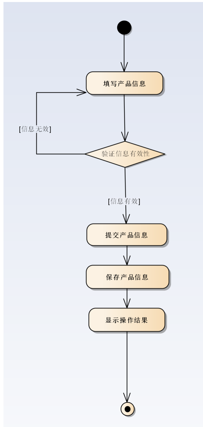
图 8.3.4 ： 产品管理 – 活动图
