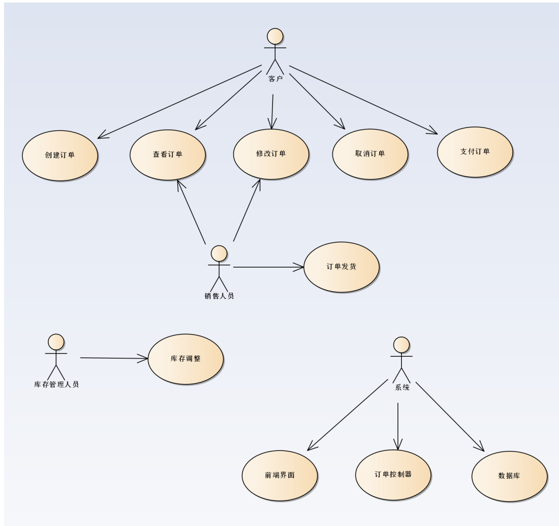
图 8.2.1 : 订单管理 – 用例图
