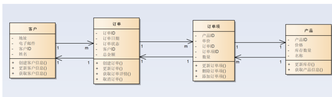
图 8.2.2 ： 订单管理 – 类图
