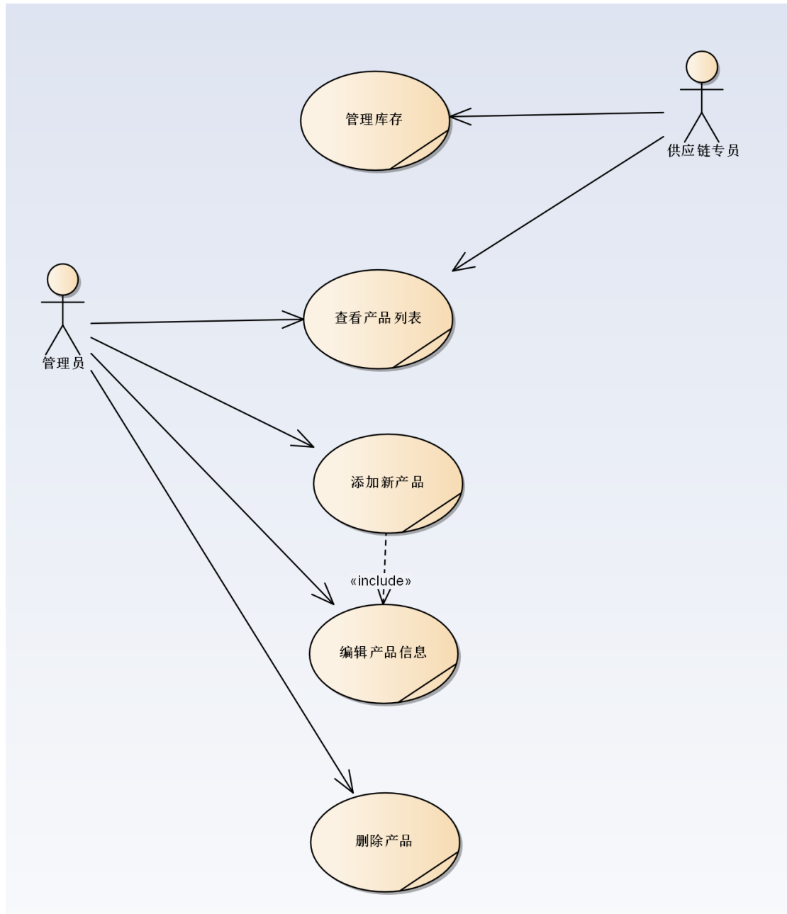
图 8.3.1 ： 产品管理 – 用例图
