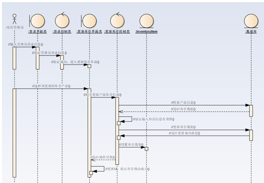
图 8.4.3 : 库存管理 – 顺序图
