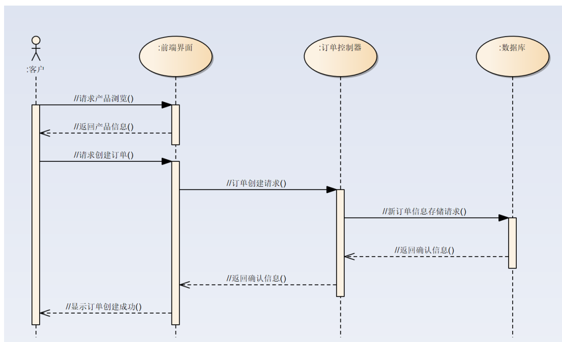
图 8.2.3 ： 订单管理 – 顺序图
