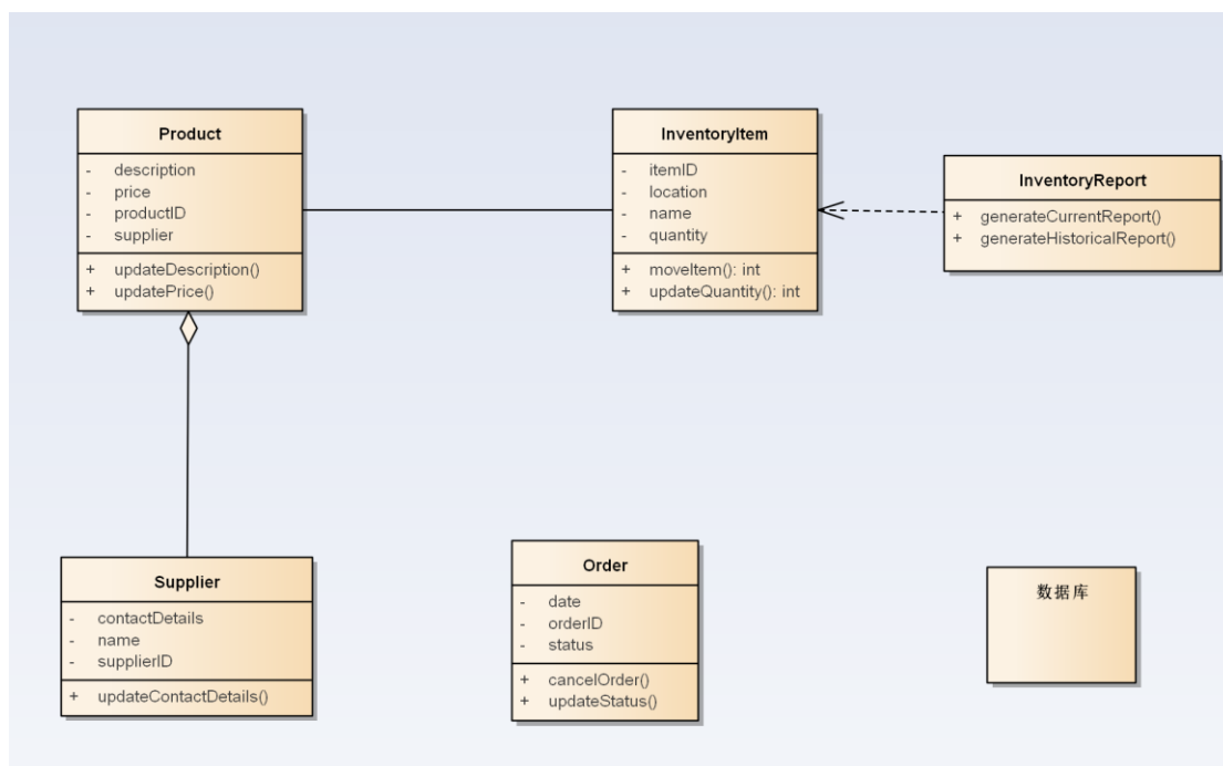
图 8.4.2：库存管理 – 类图
