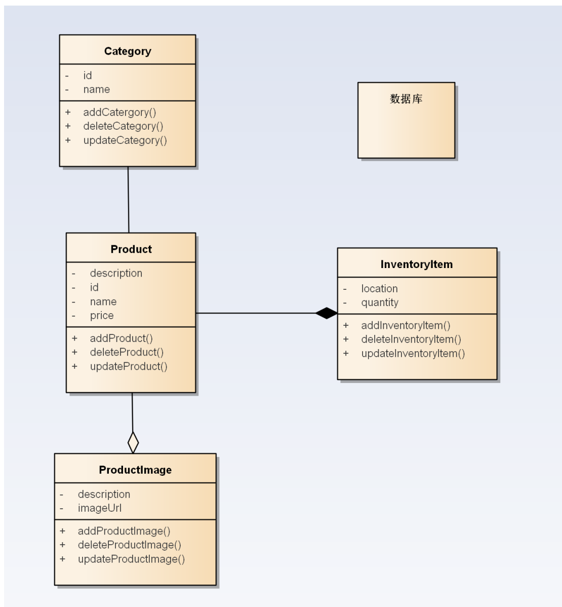
图 8.3.2：产品管理 – 类图
