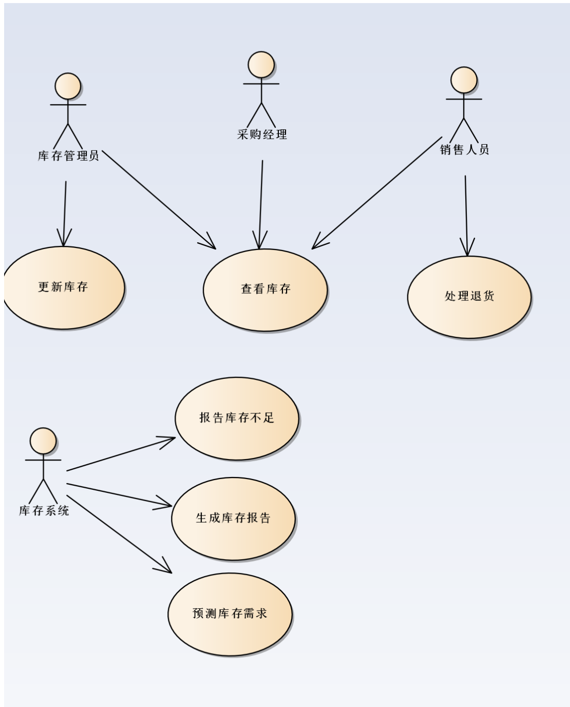
图 8.4.1 ： 库存管理 – 用例图
