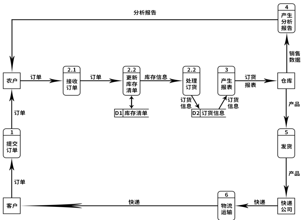
图 6.6.1.1：数据流图
