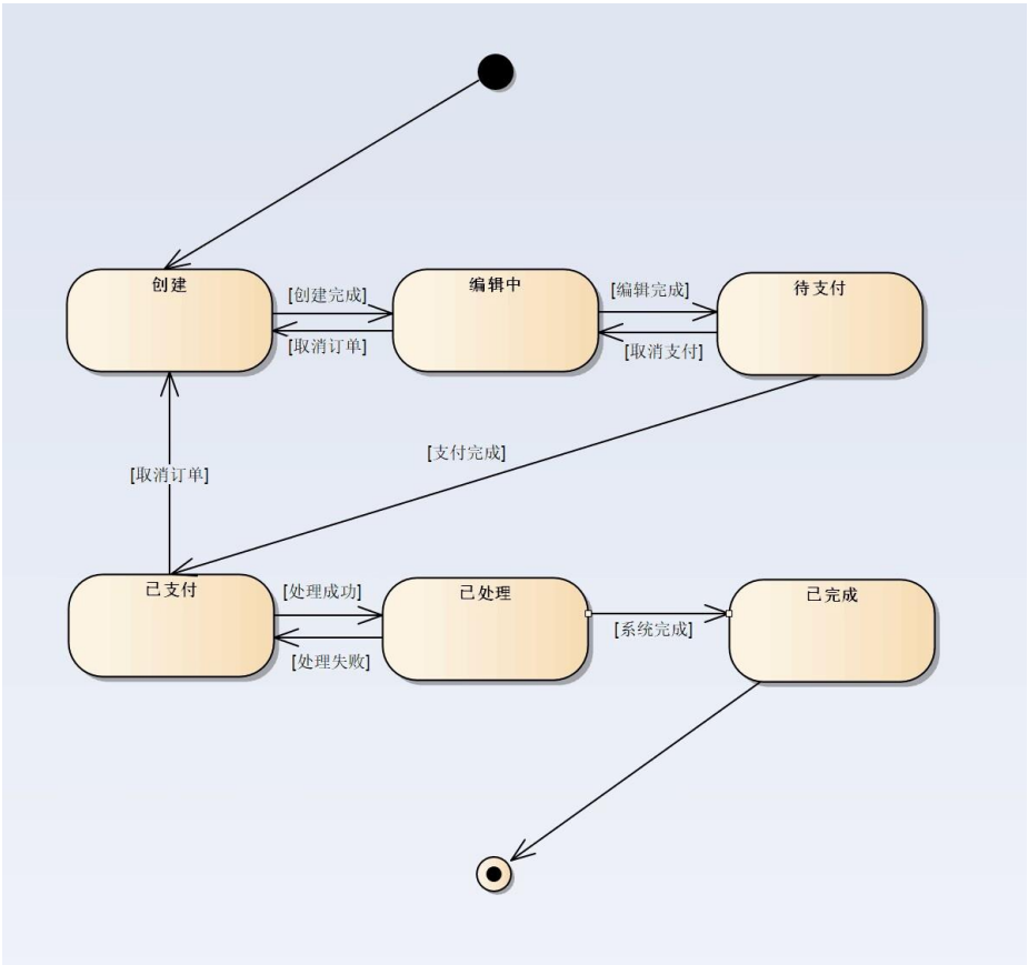
图 6.6.3.1：状态转换图
